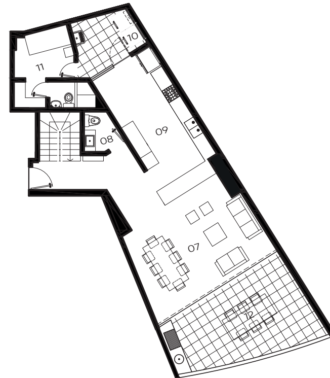
2do Nivel
